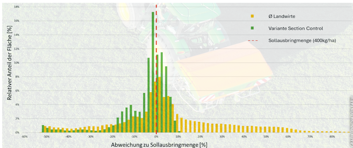
Düngemengenabweichungen mit Section Control (Variante Section Control) und ohne (Variante Landwirte)
